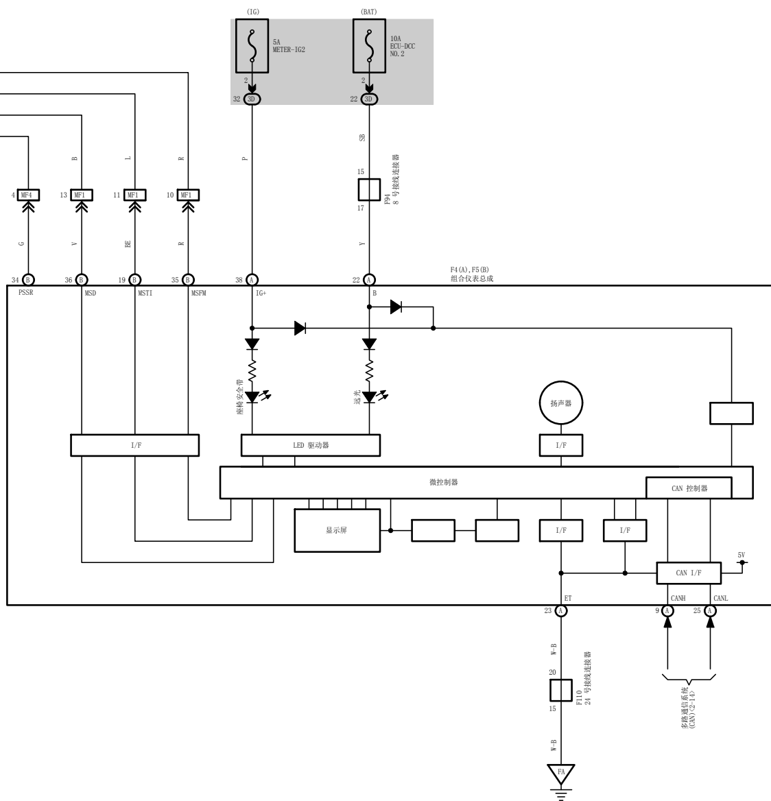
车灯提醒器
